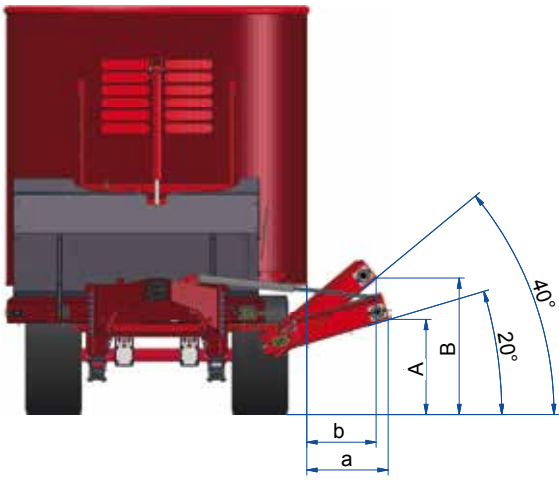
ANGLE DU TAPIS PAR RAPPORT AU SOL
