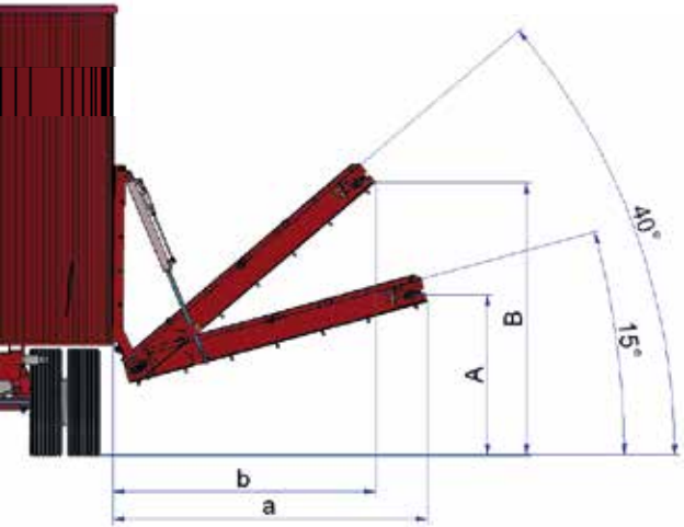
ANGLE DU TAPIS PAR RAPPORT AU SOL
